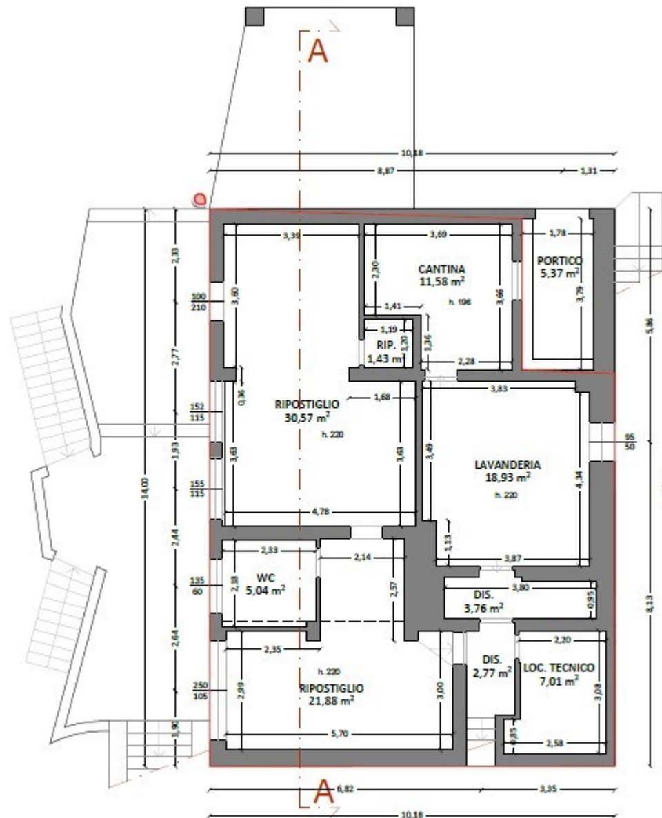
PIANTA PIANO SEMINTERRATO
